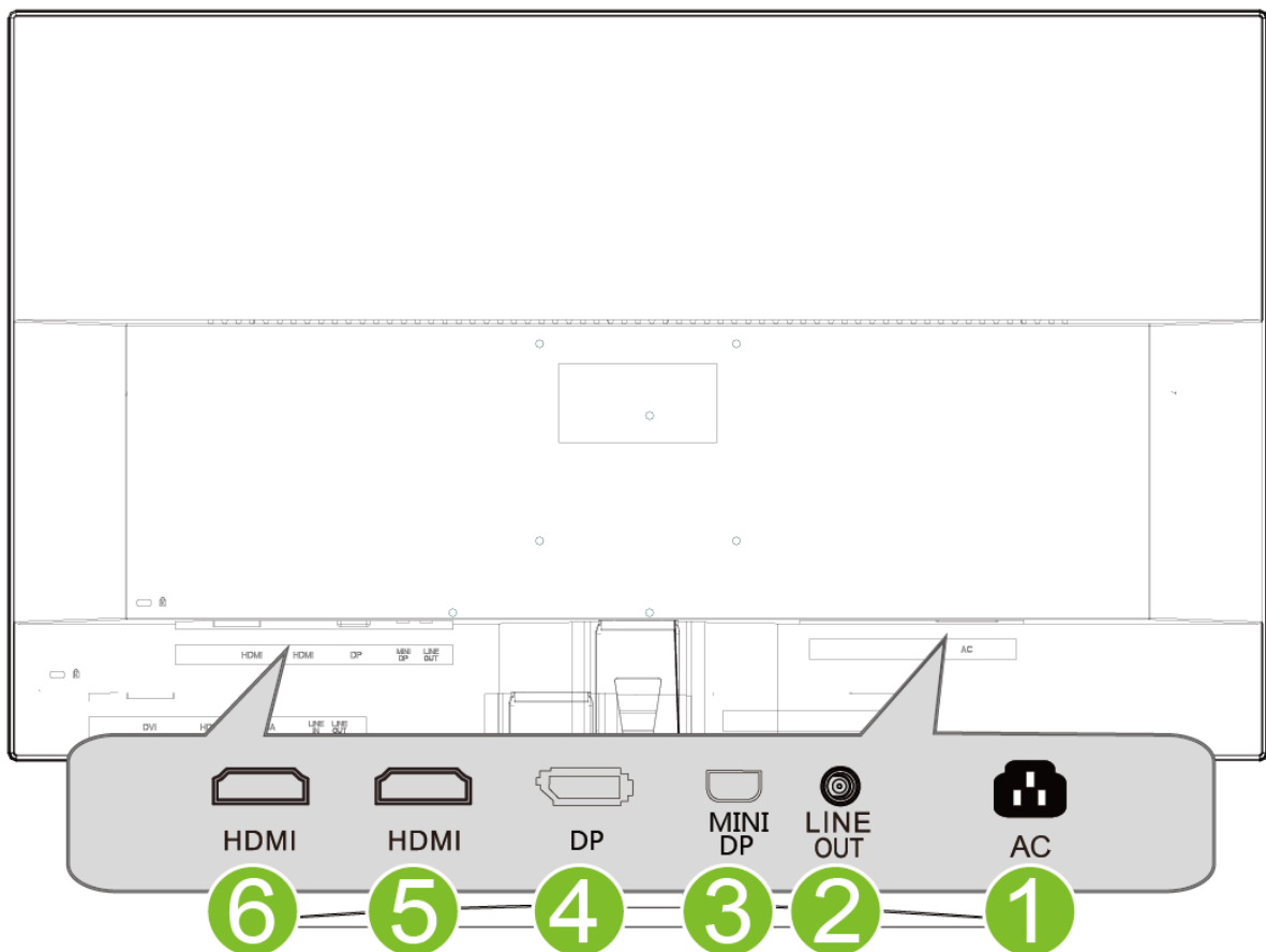
ABBILDUNG 2. ANSCHLISSEN AN EINEN PC
